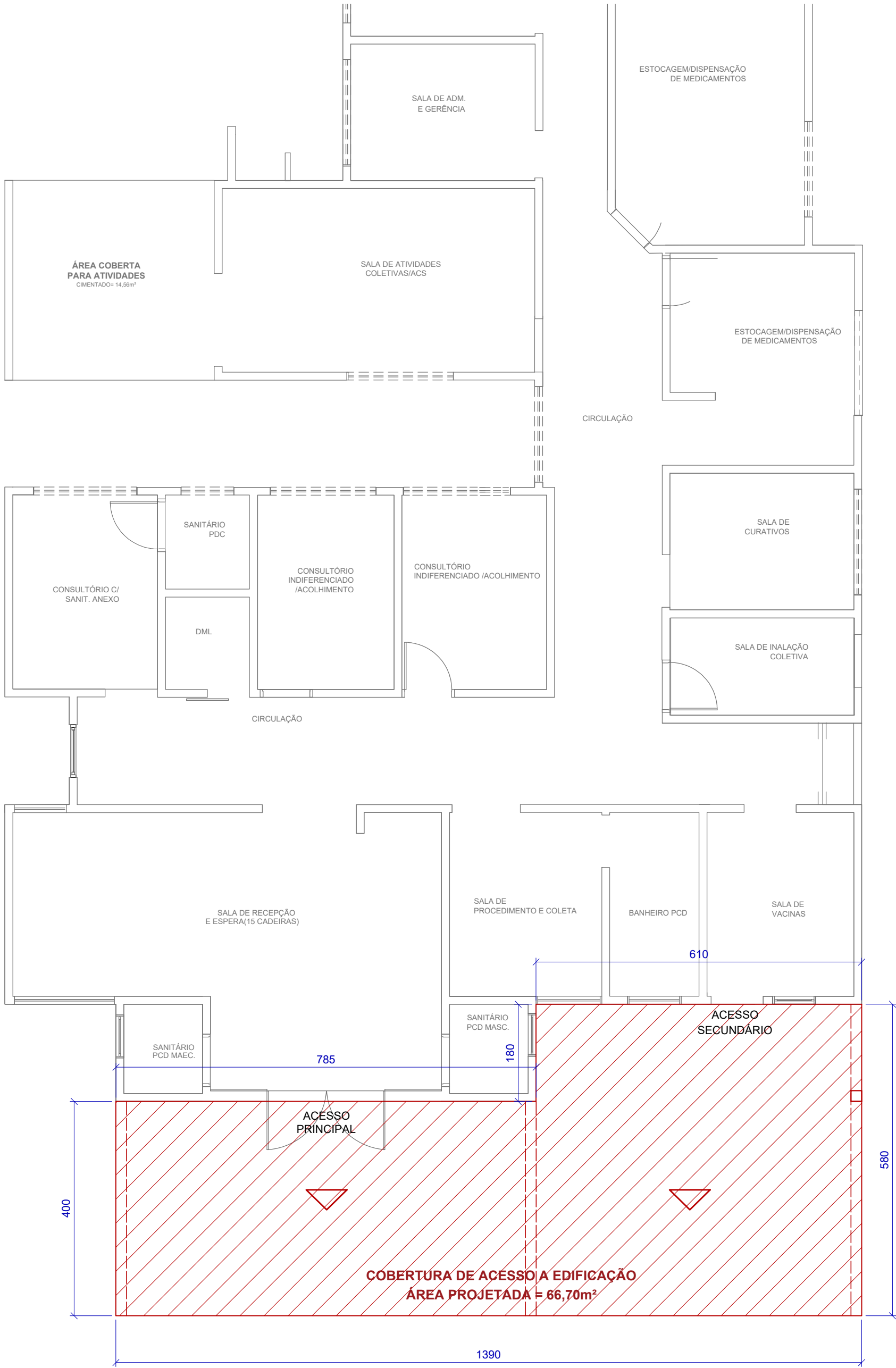
PLANTA DE IMPLANTAÇÃO ESCALA 1:75
